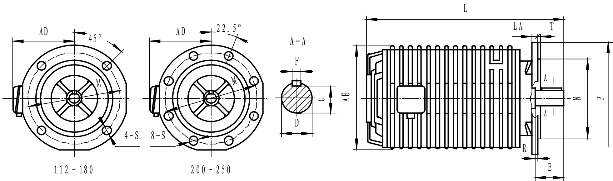
IMB5 型
