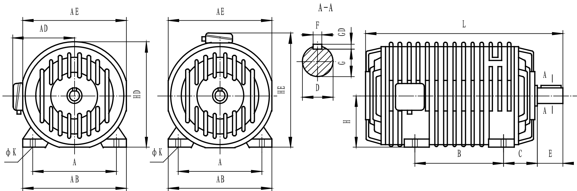
IMB3 型
